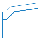
091502133 DIN 2559-3 (0°/R6/8°)
